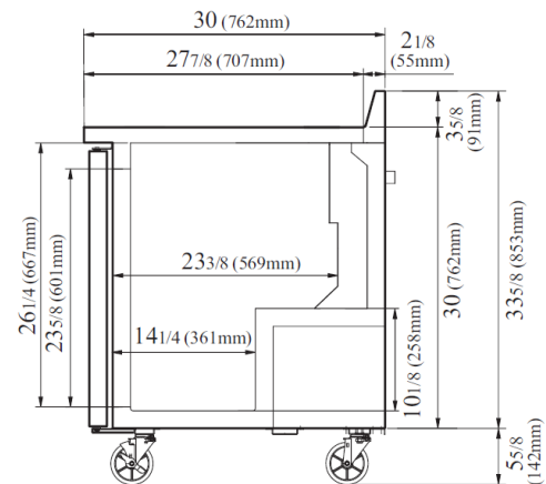
VISTA LATERAL
