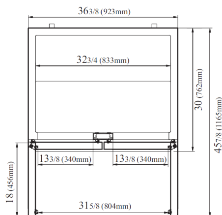
VISTA SUPERIOR
