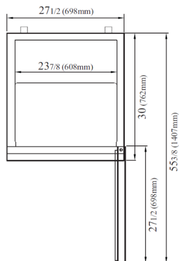
VISTA SUPERIOR
