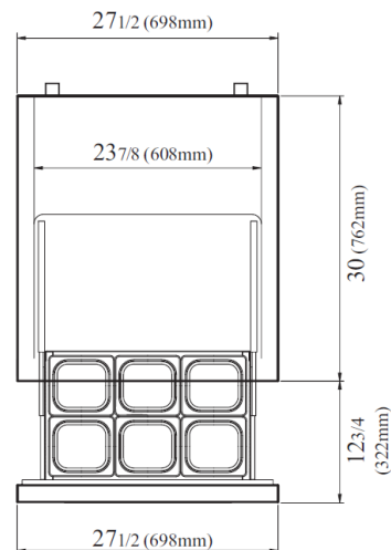
VISTA SUPERIOR
