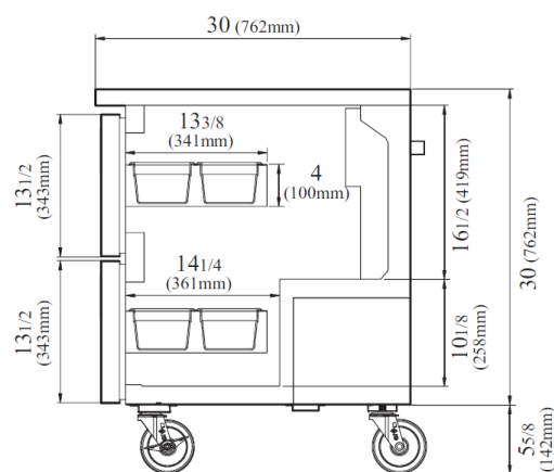
VISTA LATERAL
