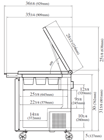
VISTA LATERAL
