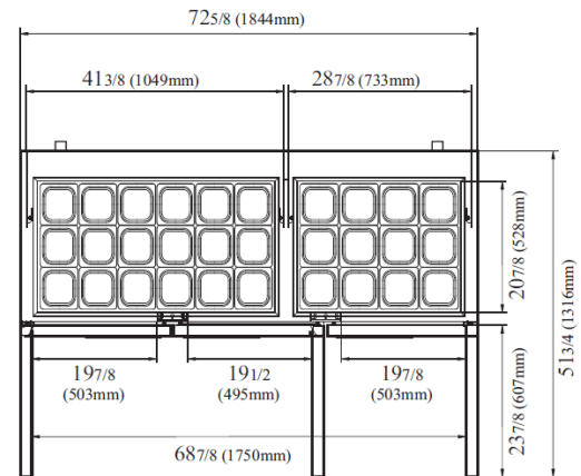
VISTA SUPERIOR
