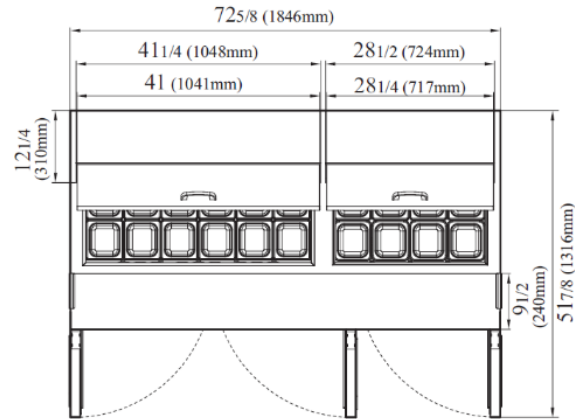
VISTA SUPERIOR
