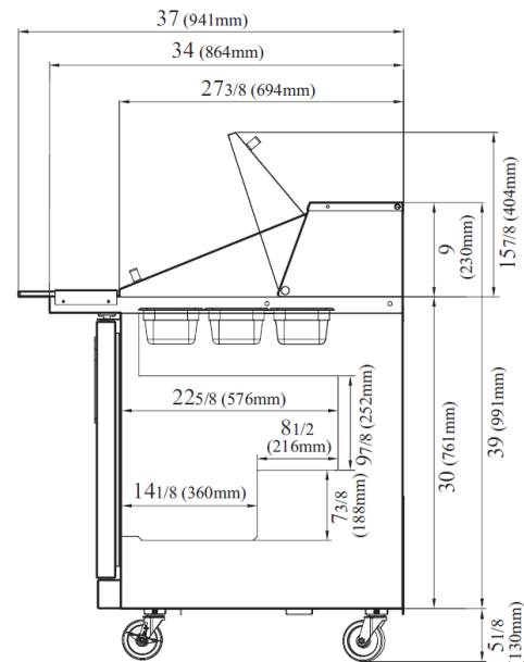
VISTA LATERAL
