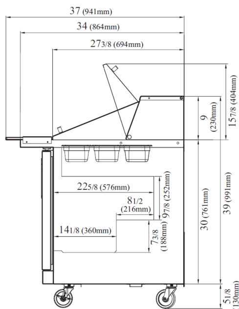
VISTA LATERAL
