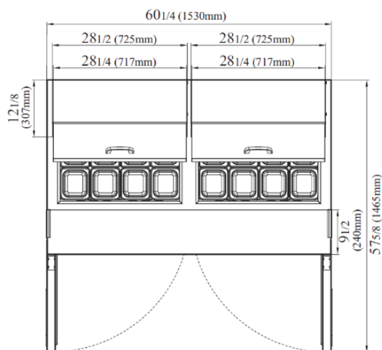
VISTA SUPERIOR
