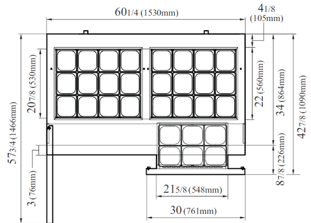
VISTA SUPERIOR
