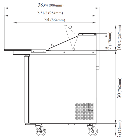
VISTA LATERAL
