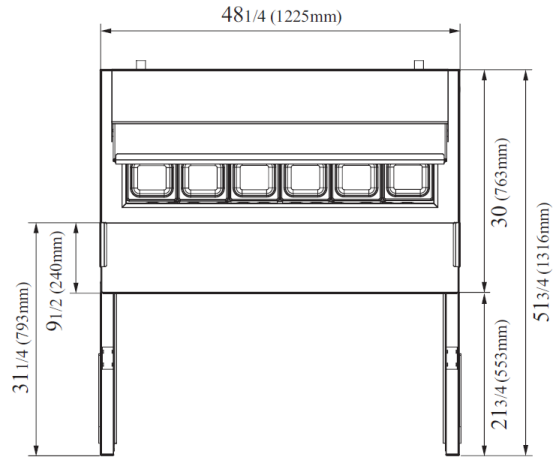
VISTA SUPERIOR
