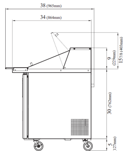
VISTA LATERAL
