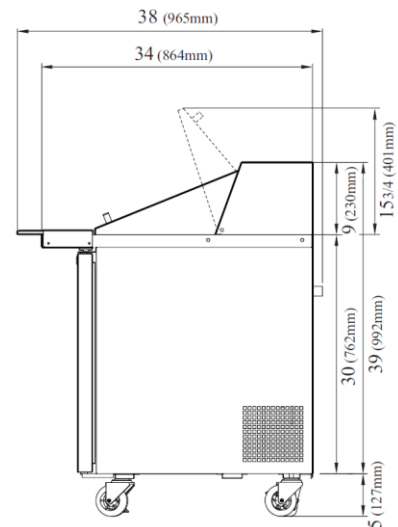
VISTA LATERAL
