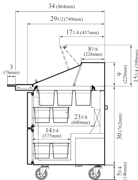
VISTA LATERAL
