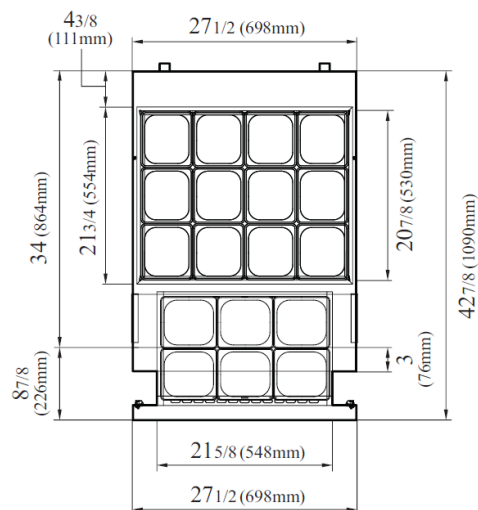
VISTA SUPERIOR
