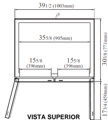
VISTA SUPERIOR
