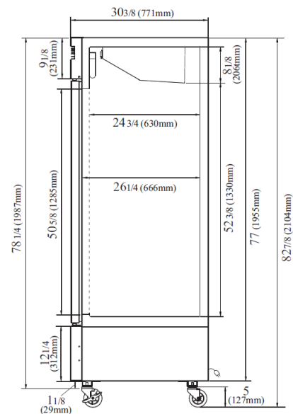
VISTA LATERAL
