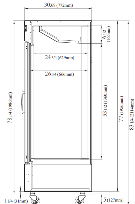
VISTA LATERAL
