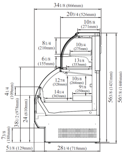
VISTA LATERAL
