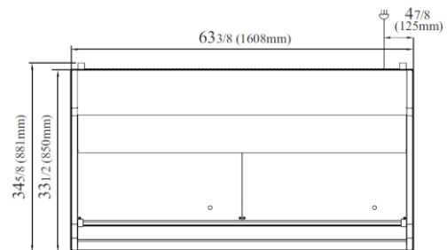
VISTA SUPERIOR
