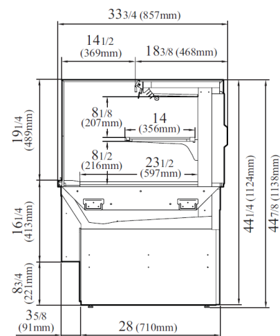
VISTA LATERAL
