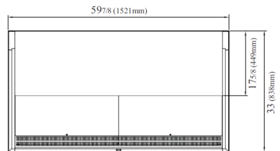
VISTA SUPERIOR
