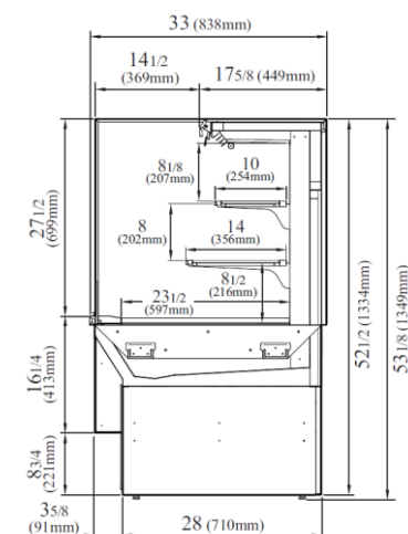
VISTA LATERAL
