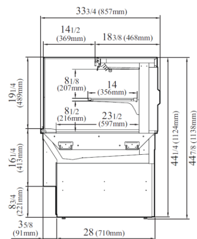
VISTA LATERAL
