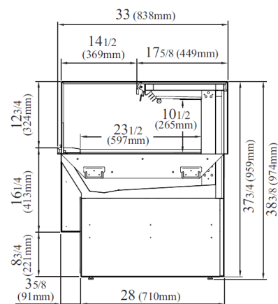
VISTA LATERAL
