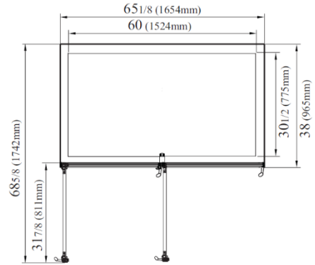
VISTA SUPERIOR
