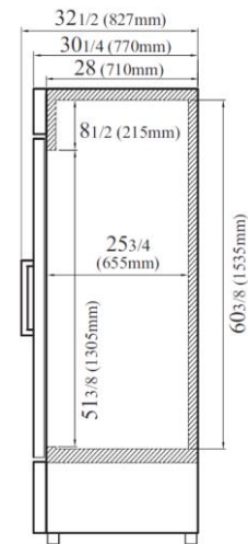
VISTA LATERAL
