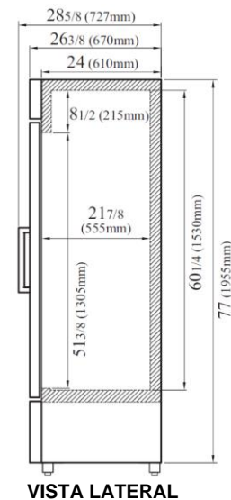
VISTA LATERAL
