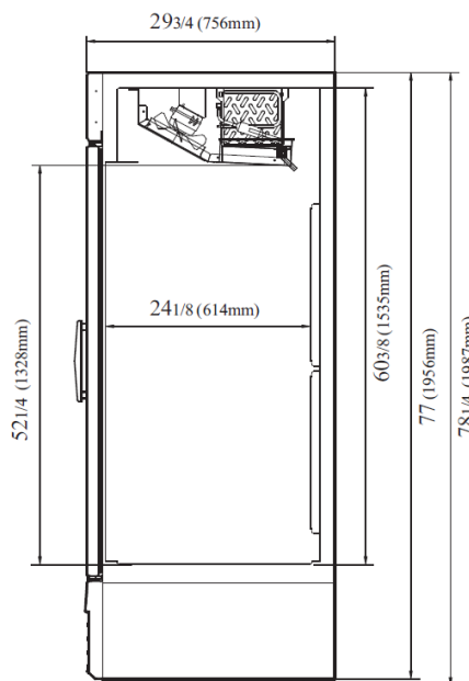
VISTA LATERAL
