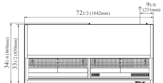
VISTA SUPERIOR
