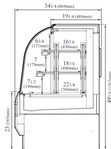
VISTA LATERAL
