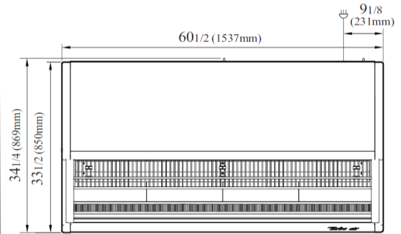
VISTA SUPERIOR
