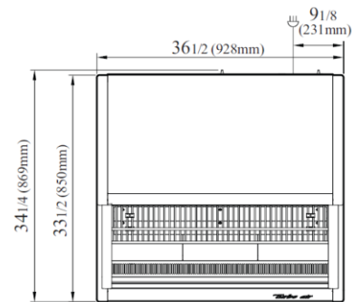
VISTA SUPERIOR
