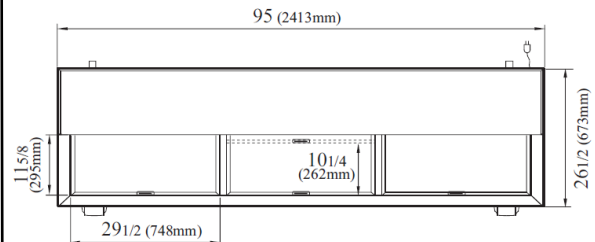
VISTA SUPERIOR
