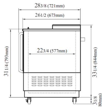
VISTA LATERAL
