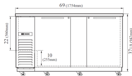
TBB-3SBD-N6 VISTA FRONTAL
