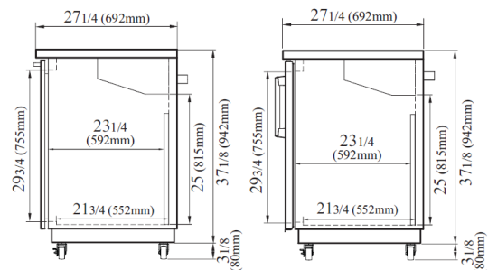
TBB-3SBD-N6 Y TBB-3SGD-N VISTA LATERAL
