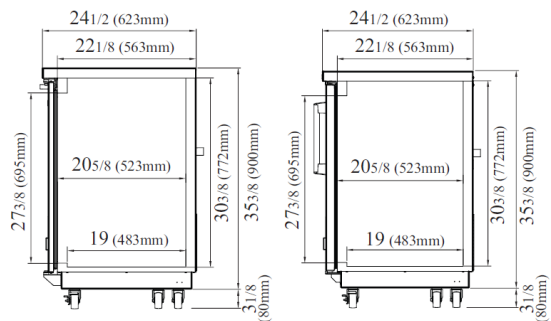
TBB-24-48SSD-N6 Y TBB-24-48SGSD-N VISTA LATERAL
