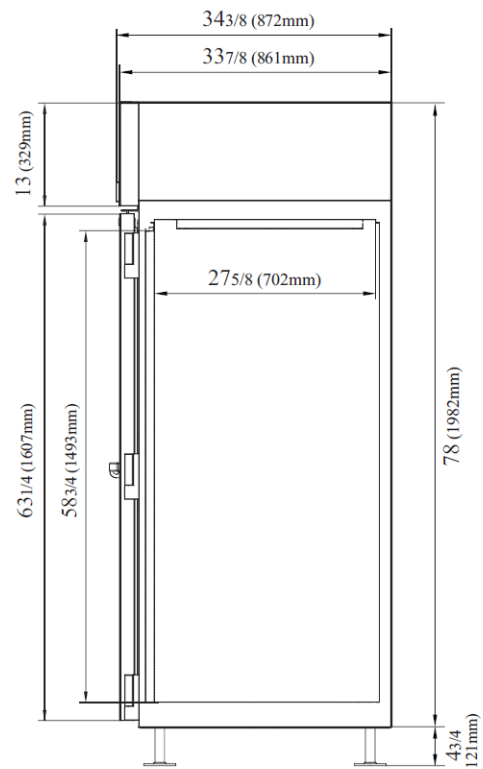
VISTA LATERAL
