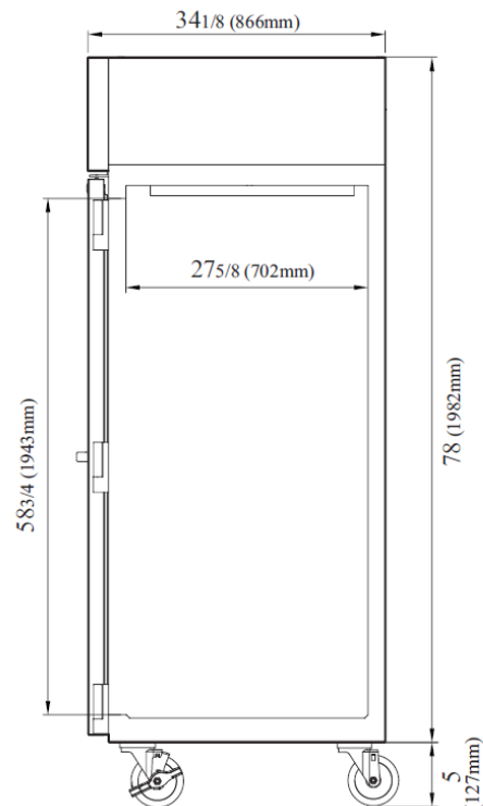
VISTA LATERAL
