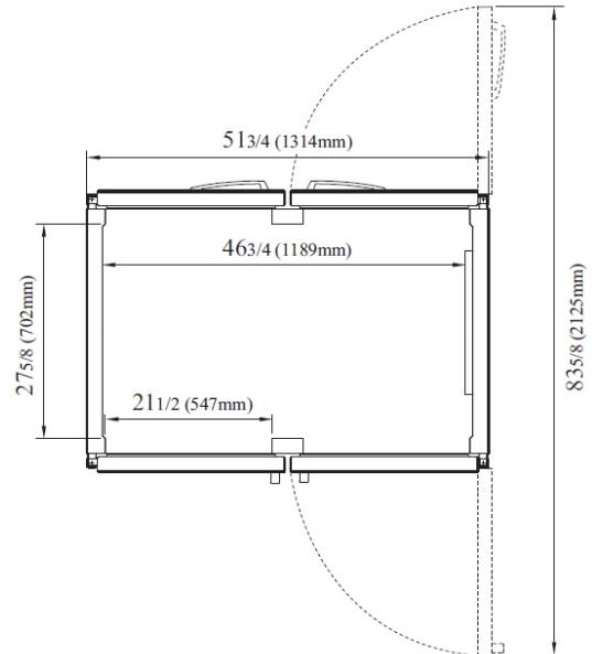
VISTA SUPERIOR
