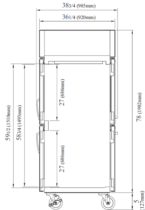
VISTA LATERAL
