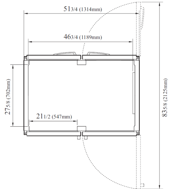
VISTA SUPERIOR
