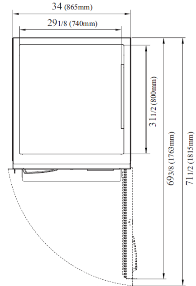
VISTA SUPERIOR
