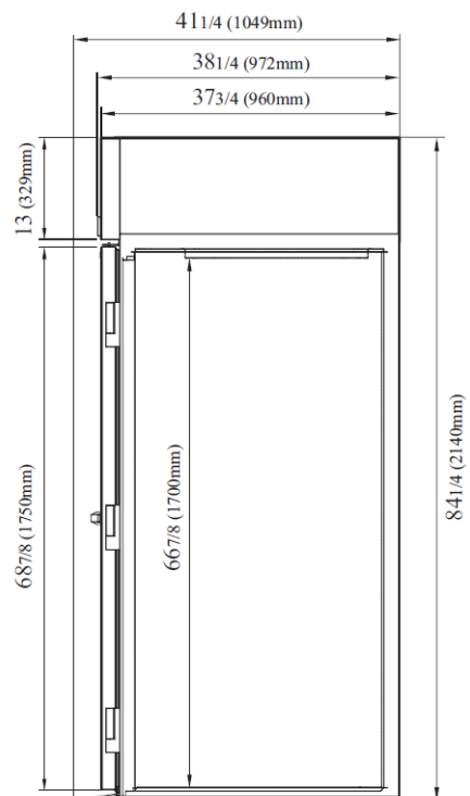
VISTA LATERAL
