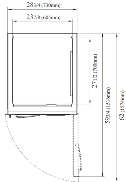
VISTA SUPERIOR
