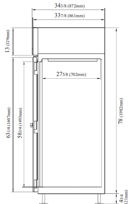
VISTA LATERAL
