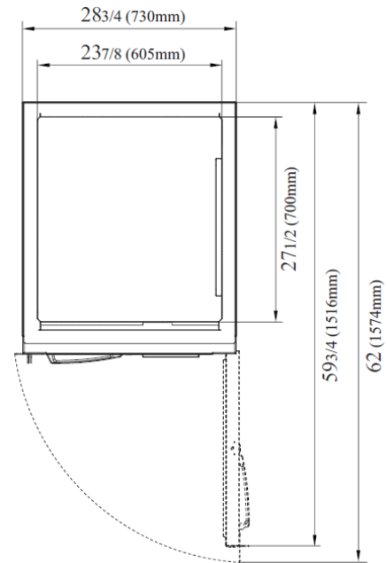
VISTA SUPERIOR
