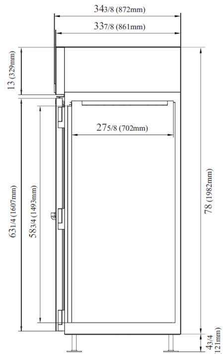
VISTA LATERAL
