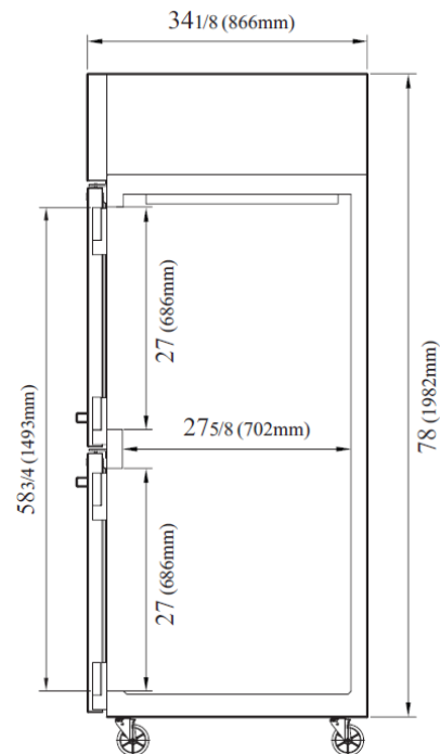
VISTA LATERAL
