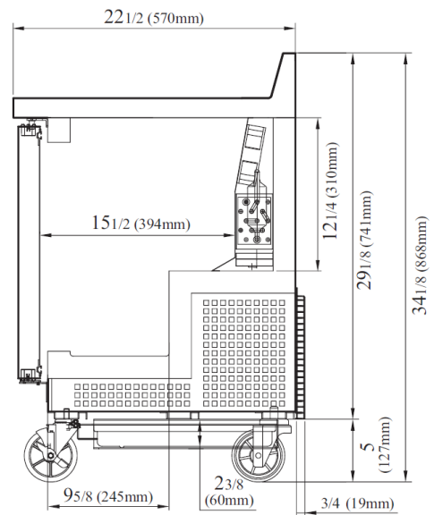
VISTA LATERAL
