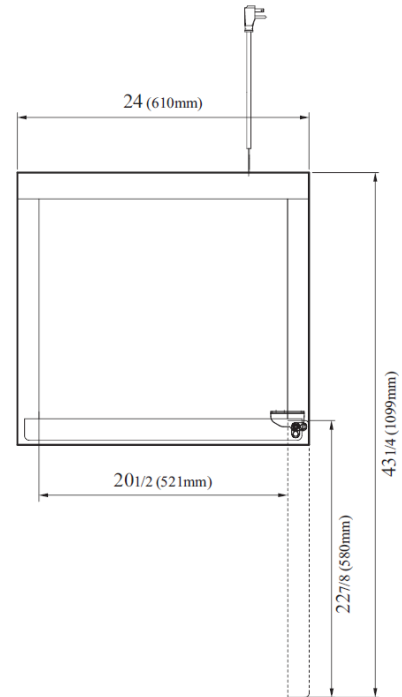
VISTA SUPERIOR
