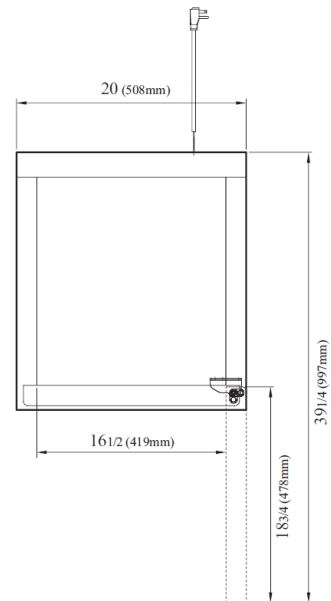
VISTA SUPERIOR
