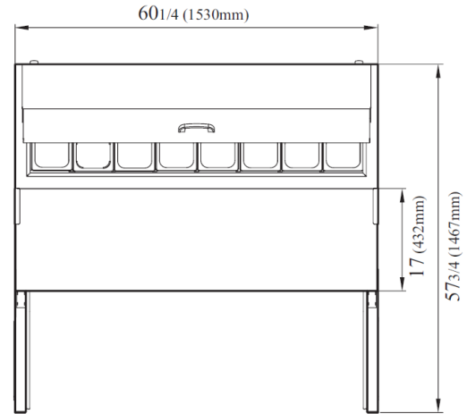
VISTA SUPERIOR
