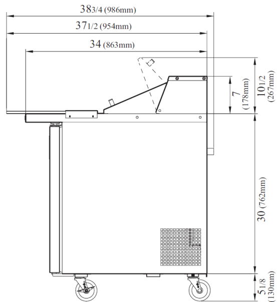
VISTA LATERAL
