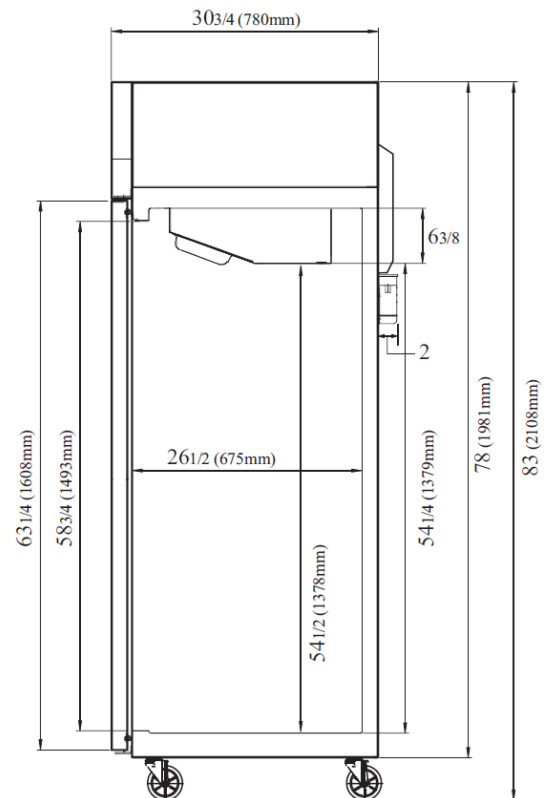
VISTA LATERAL
