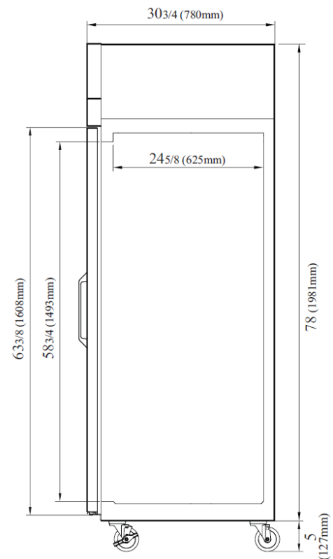
VISTA LATERAL
