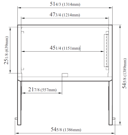
VISTA SUPERIOR
