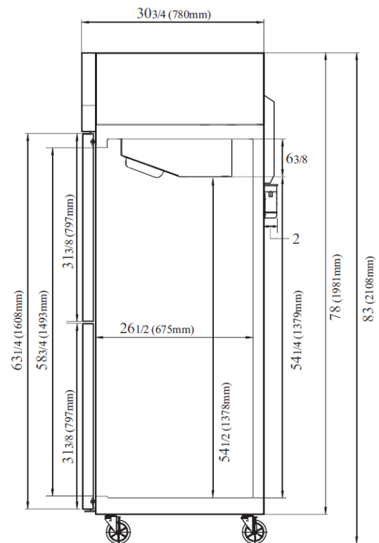
VISTA LATERAL
